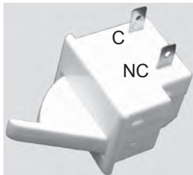
Refrigerator Door Switch
